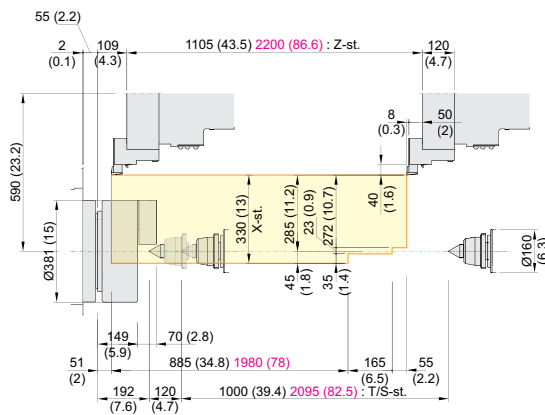
O.D Tool
