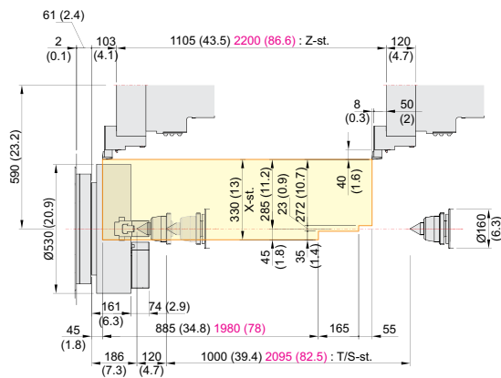
O.D Tool
